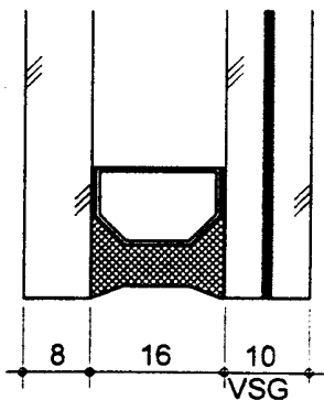
Bild 1 Schnitt durch den Probekörper
